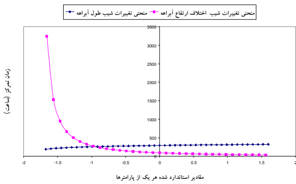
شکل 6. نمودار تغییرات شیب متغیر های رابطه کالیفرنیا
