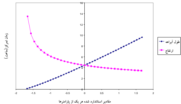
شکل 1. نمودار آنالیز حساسیت متغیرهای رابطه کالیفرنیا
