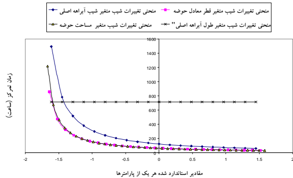
شکل 7. نمودار تغییرات شیب متغیر های رابطه برانسلی-ویلیامز
