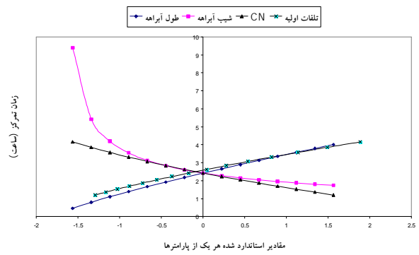
شکل 3. نمودار آنالیز حساسیت متغیر های رابطه SCS
