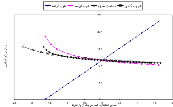
شکل 4. نمودار آنالیز حساسیت متغیر های رابطه برانسلی-ویلیامز
