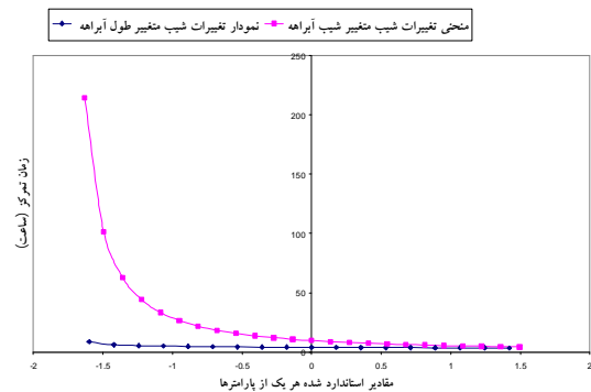
شکل 5. نمودار تغییرات شیب متغیر های رابطه کرپیچ
