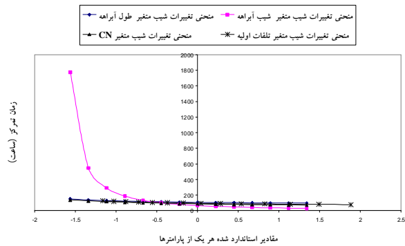
شکل 8. نمودار تغییرات شیب متغیر های رابطه SCS
