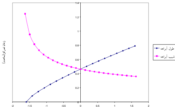
شکل 2. نمودار آنالیز حساسیت متغیرهای رابطه کرپیچ
