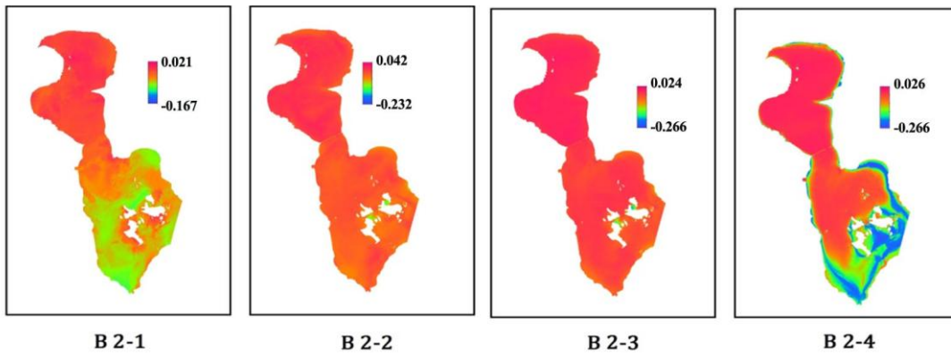
شکل ۸. تغییرات طیفی باند ۲ تصاویر TM و باندهای مشابه (باند ۲ها) در گستره زمانی مورد مطالعه.
