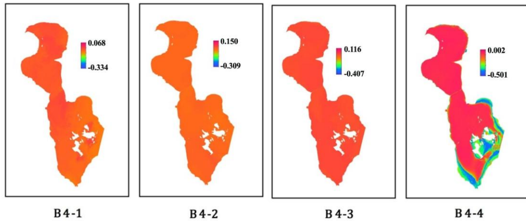
شکل ۱۰. تغییرات طیفی باند ۴ تصاویر TM و باندهای مشابه (باند ۴ها) در گستره زمانی مورد مطالعه.
