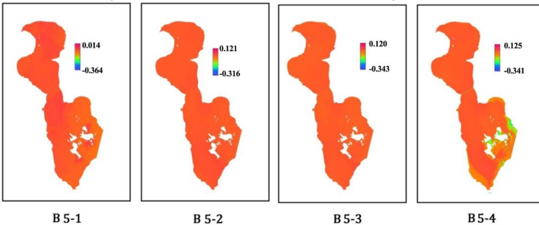
شکل ۱۱. تغییرات طیفی باند ۵ تصاویر TM و باندهای مشابه (باند ۵ها) در گستره زمانی مورد مطالعه.
