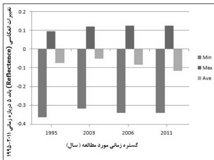
شکل ۶. میزان تغییرات انعکاس طیفی بین باندهای ۵ گستره زمانی بیانگر تغییر گستره آبی دریاچه ارومیه.
