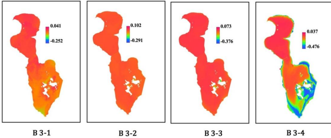
شکل ۹. تغییرات طیفی باند ۳ تصاویر TM و باندهای مشابه (باند ۳ها) در گستره زمانی مورد مطالعه.
