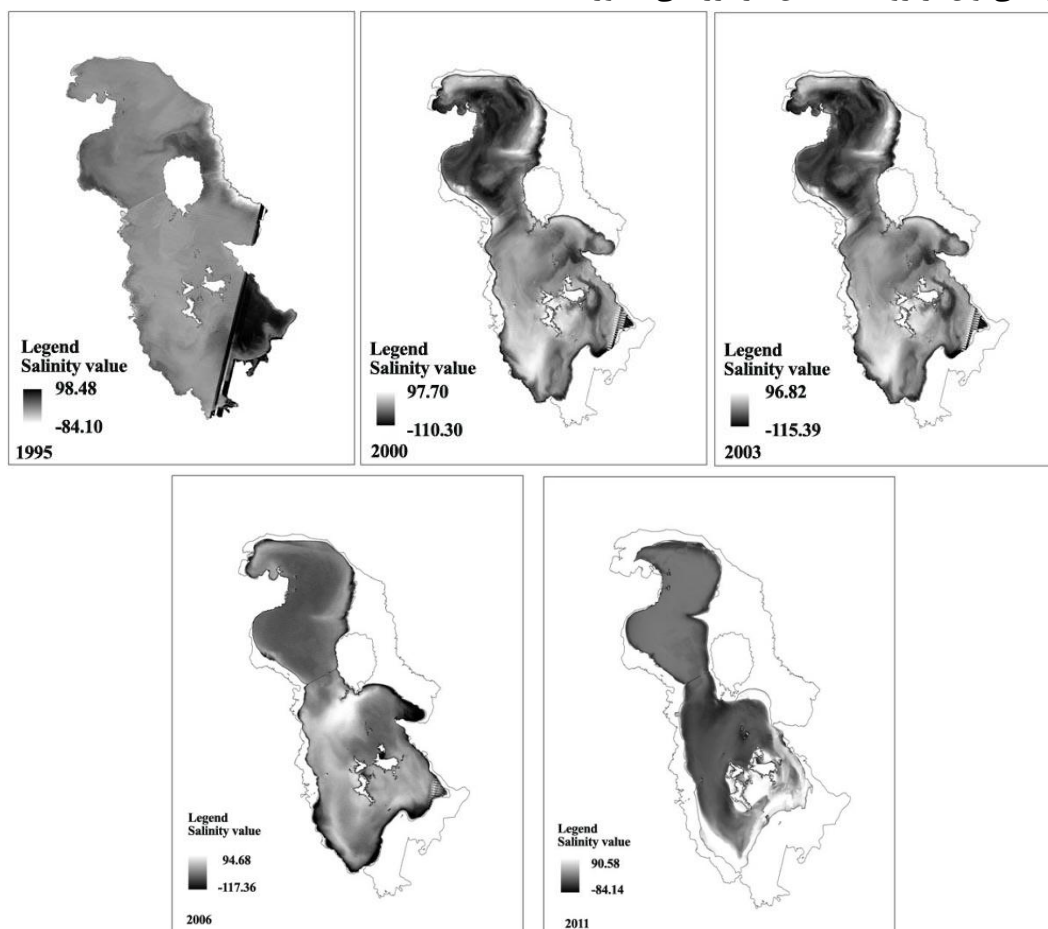
شکل ۱۲. مدل پراکنش و تغییرات میزان شوری دریاچه ارومیه.
