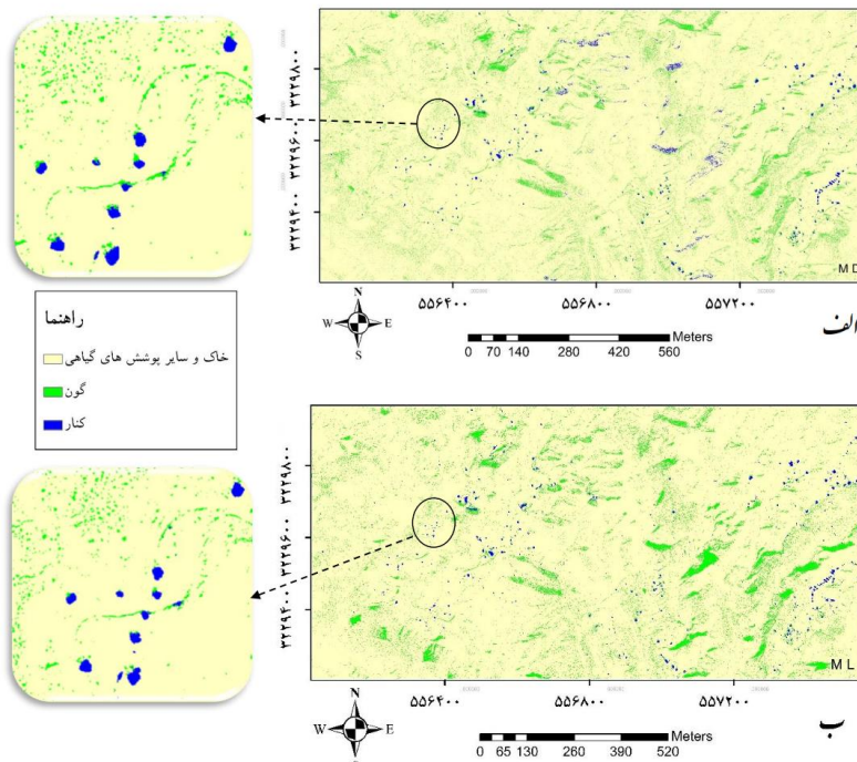
شکل ۳- طبقه‌بندی گروه هفت باندی (چهار باند اصلی، NDVI، PC1 و SAVI) با الگوریتم‌های پارامتری الف) حداکثر احتمال و ب) فاصله ماله‌انویسی
