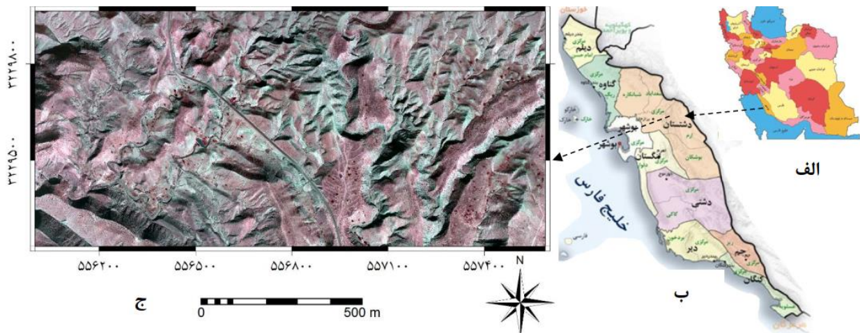
شکل ۱- موقعیت محدوده مورد مطالعه در الف) ایران، ب) استان بوشهر و ج) تصویر UC-D با ترکیب باندی ۳، ۴ و ۲
