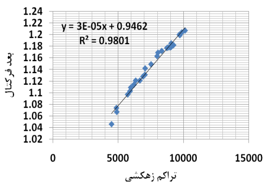
شکل ۶- رگرسیون خطی بین بعد فراکتال و دو شاخص تراکم‌زهکشی و رتبه آبراهه (سازند تفت)
