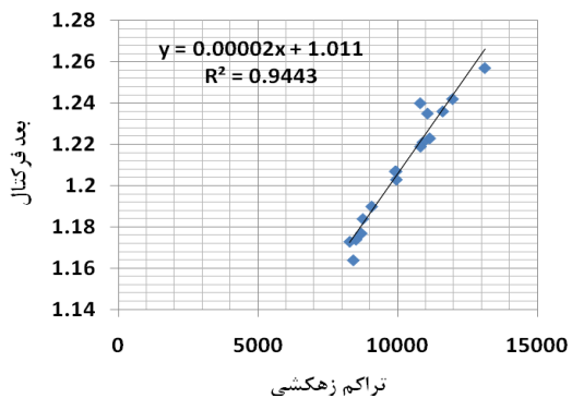
شکل ۸- رگرسیون خطی بین بعد فراکتال و دو شاخص تراکم‌زهکشی و رتبه آبراهه (سازند کهر)
