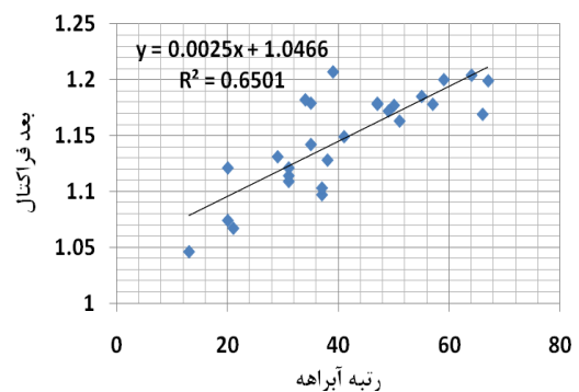
شکل ۶- رگرسیون خطی بین بعد فراکتال و دو شاخص تراکم‌زهکشی و رتبه آبراهه (سازند تفت)
