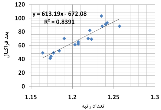
شکل ۸- رگرسیون خطی بین بعد فراکتال و دو شاخص تراکم‌زهکشی و رتبه آبراهه (سازند کهر)
