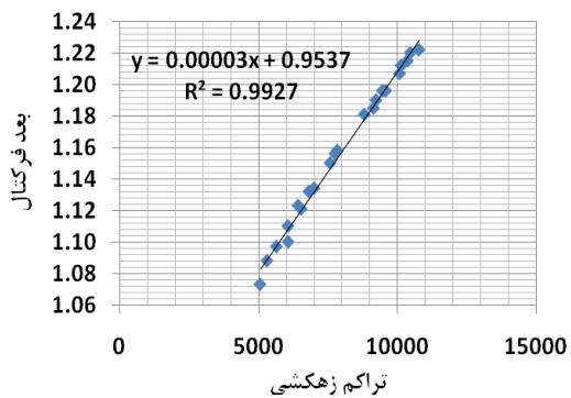
شکل ۷- رگرسیون خطی بین بعد فراکتال و دو شاخص تراکم‌زهکشی و رتبه آبراهه (سازند گرانیت شیرکوه)
