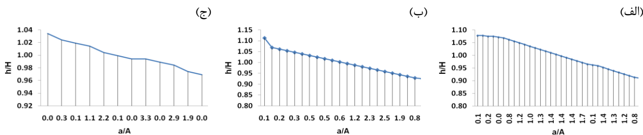
شکل ۵- شاخص انتگرال هیپسومتری HI الف) سازند آهک تفت ب) سازند گرانیت ج) سازند کهر
