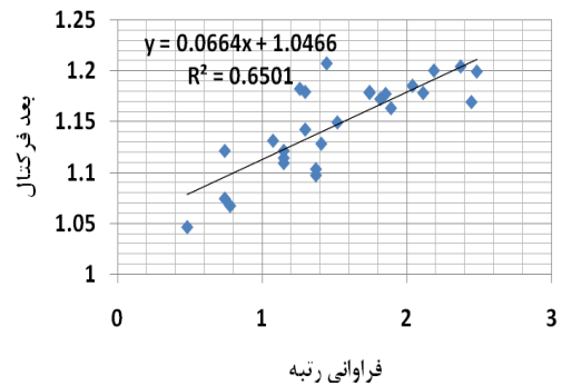
شکل ۹- رگرسیون خطی بین بعد فراکتال و دو شاخص فراوانی رتبه و متوسط طول رتبه (سازند تفت)
