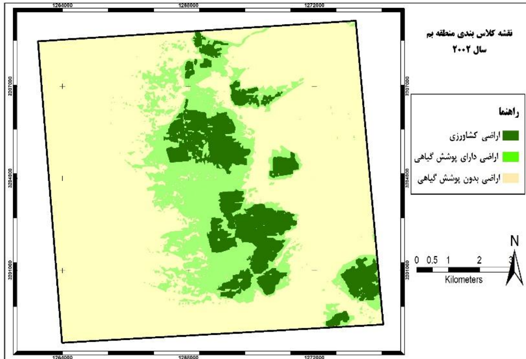
شکل ۳- نقشه کاربری اراضی استخراج‌شده از تصویر لندست سال ۲۰۰۲ منطقه بم
