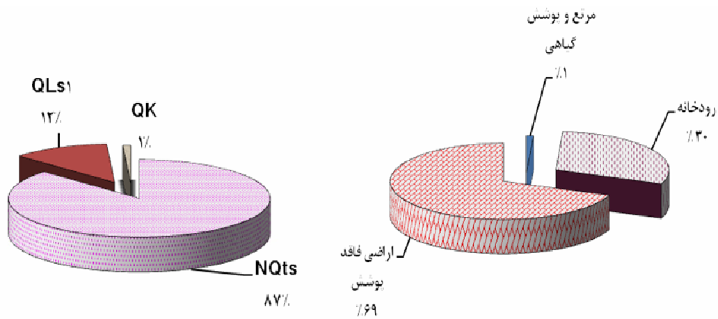
شکل 2. مقایسه سهم رسوب منابع رسوب
