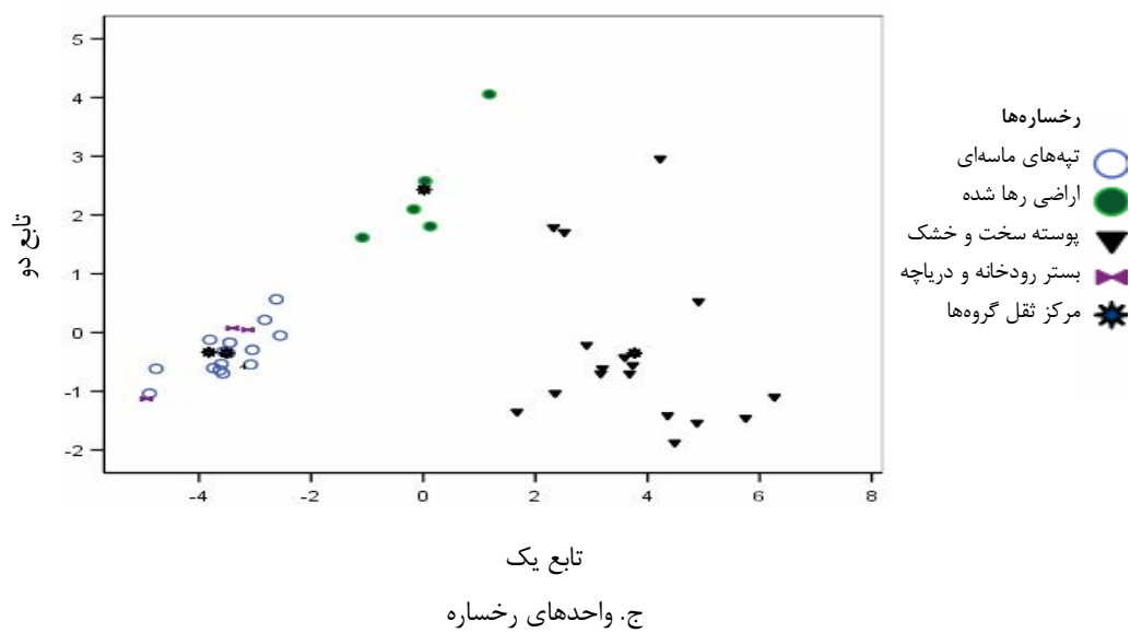
شکل 1. نمودار پراکنش تابع 1 در مقابل تابع 2 در تفکیک منابع رسوب
