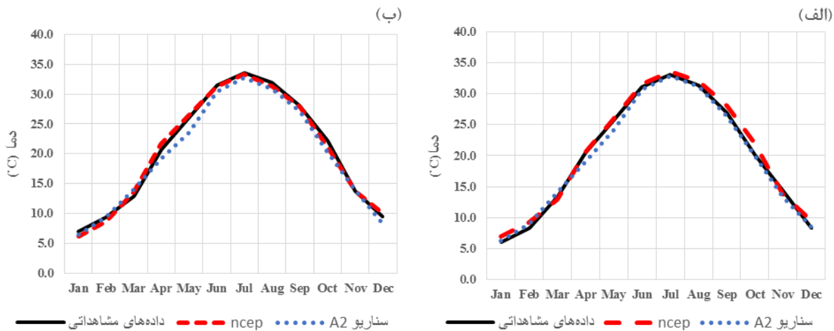
شکل ۱۴- مقایسه دمای میانگین ماهانه مشاهداتی و شبیه‌سازی شده توسط مدل SDSM در دو دوره واسنجی ۱۹۸۷-۱۹۹۷
