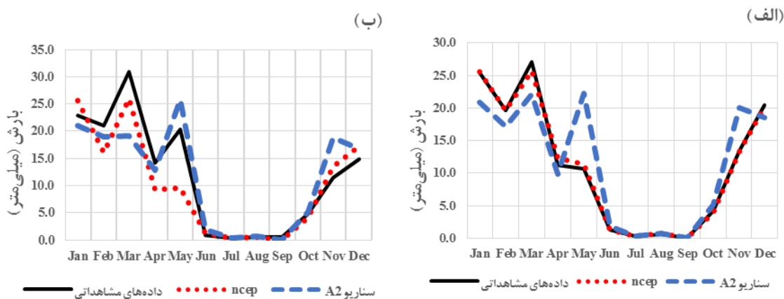
شکل ۲- مقایسه بارش میانگین ماهانه مشاهداتی و شبیه‌سازی شده توسط مدل SDSM در دو دوره واسنجی ۱۹۷۱-۱۹۹۱ (الف) و صحت‌سنجی ۲۰۰۱-۱۹۹۲ (ب) ایستگاه کاشان
